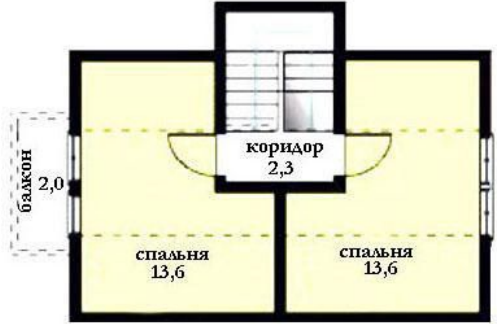
План мансарды
